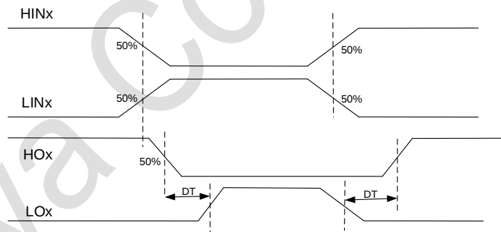
图 5-8 死区功能
