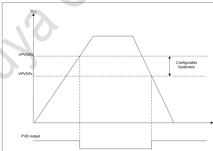
图 2-4 PVD 阈值
