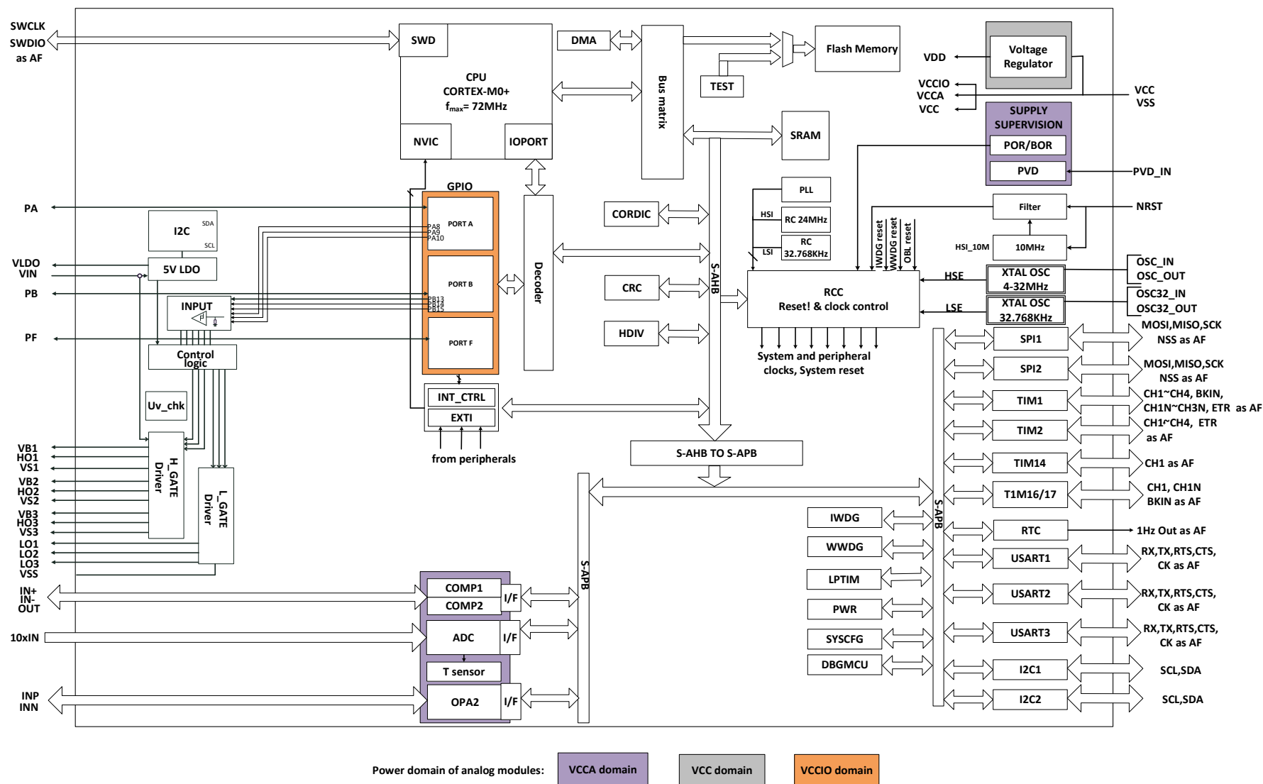
图 1-1 LQFP48/QFN40 功能模块
