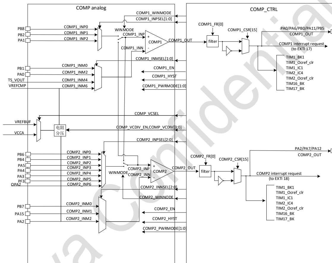
图 2-5 COMP 框图
