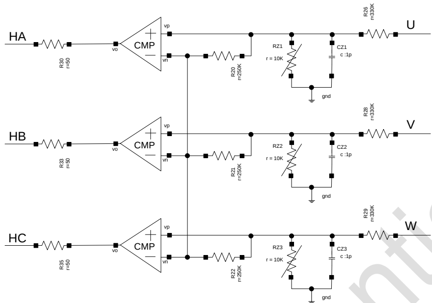
图 5-15 过零检测内部电路框图
