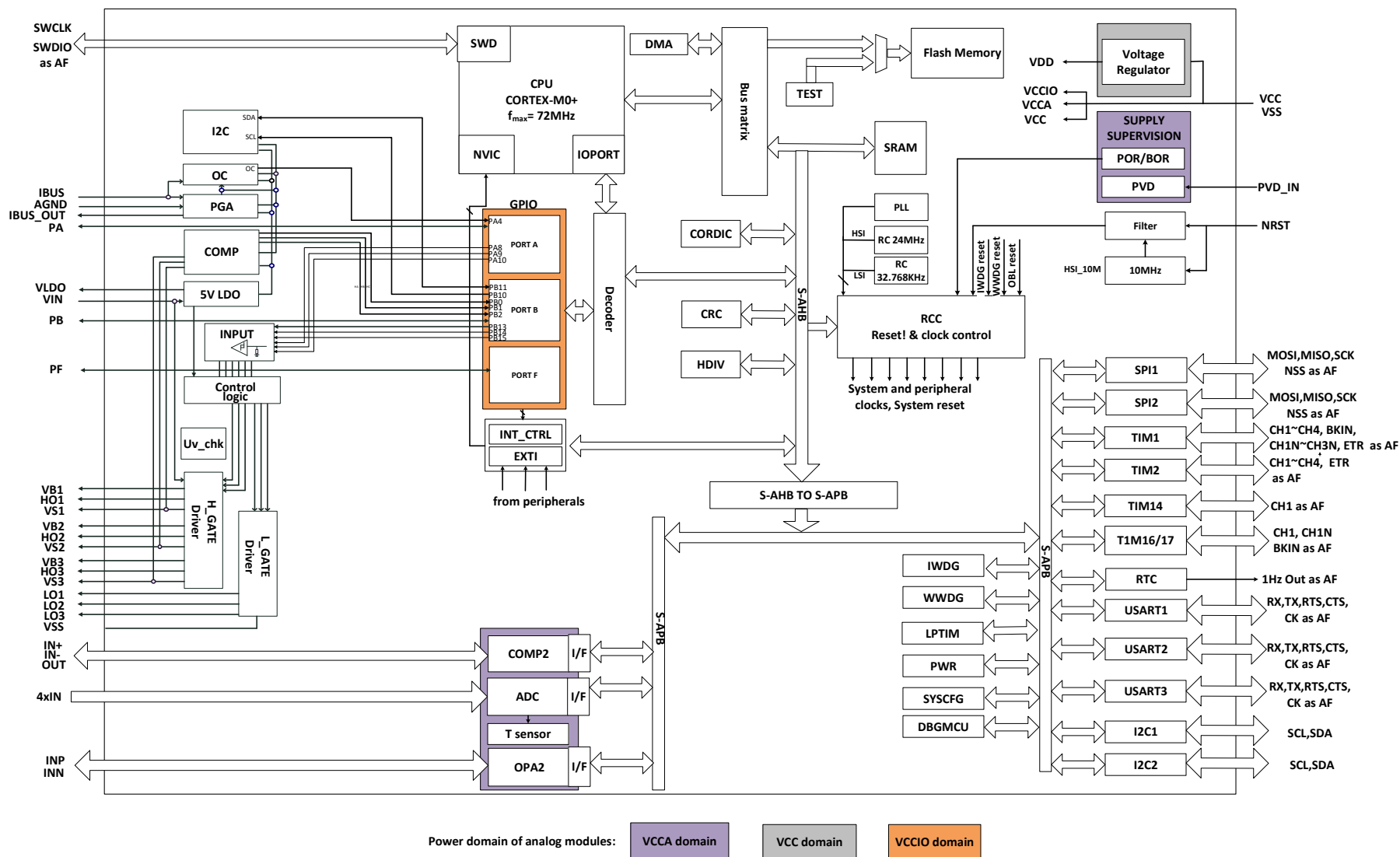
图 1-2 QFN32 功能模块
