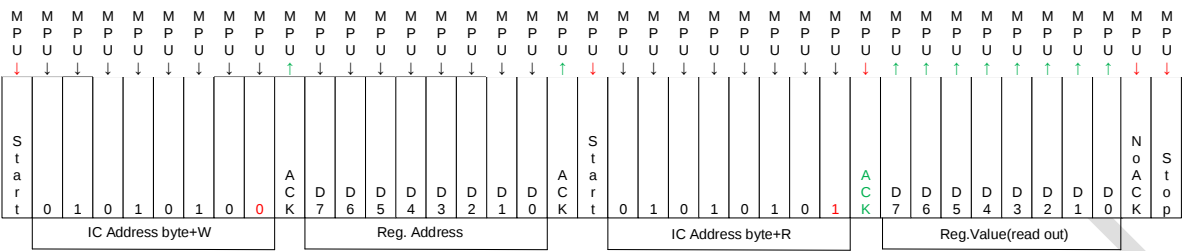
图 5-14 读命令格式
