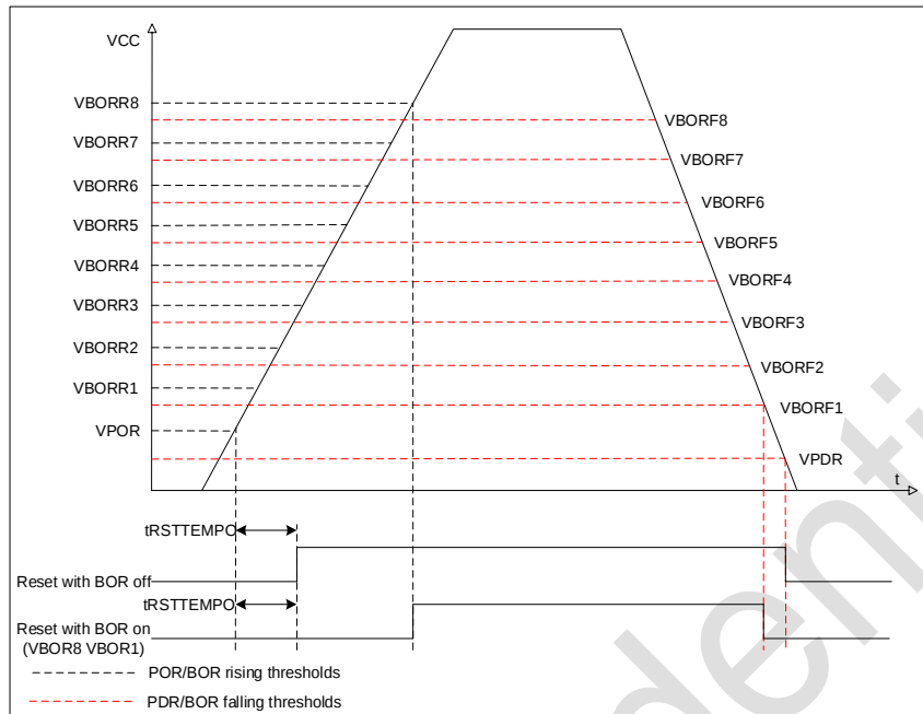
图 2-3 POR/PDR/BOR 阈值
