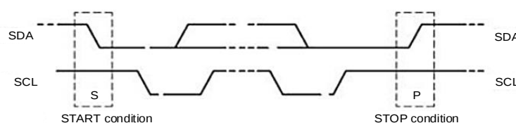
图 5-9 起始和停止条件
