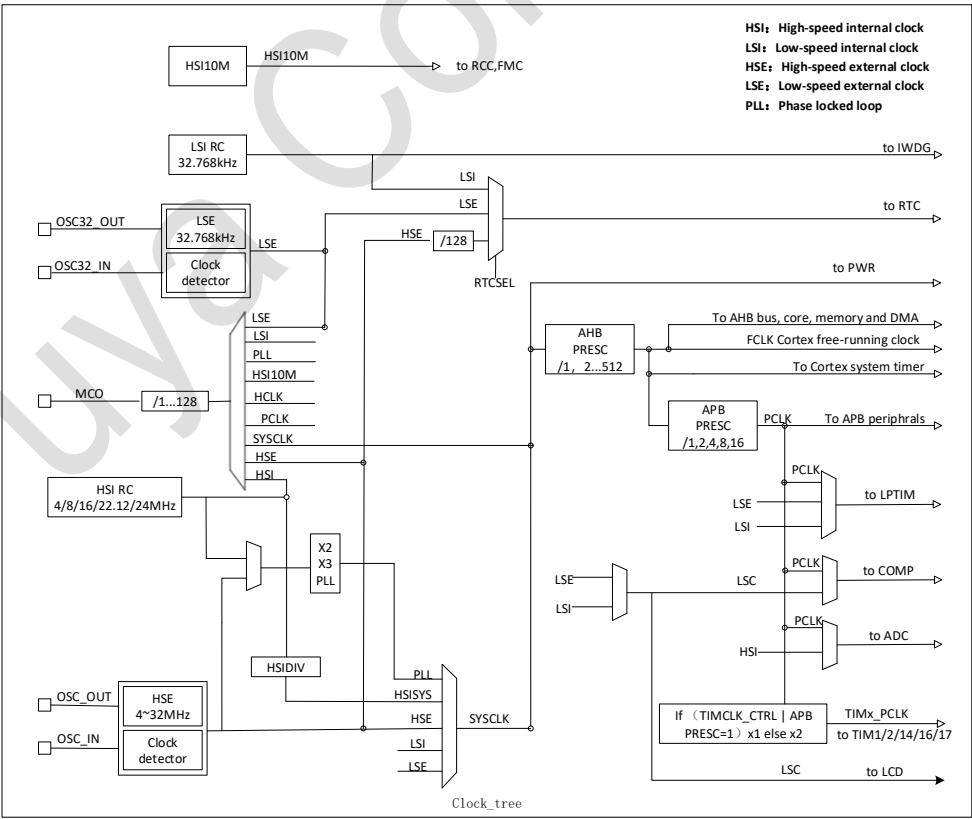
图 2-1 系统时钟结构图
