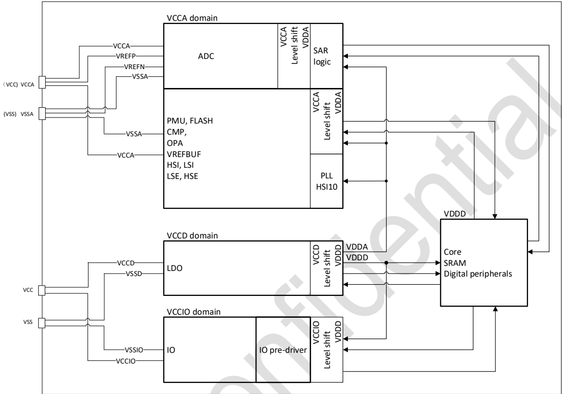
图 2-2 电源框图
